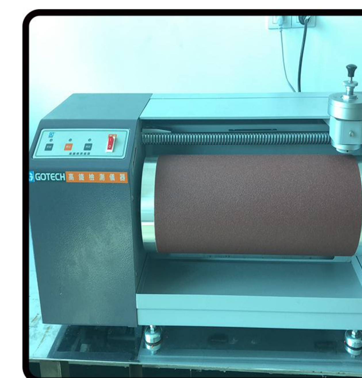
DIN ABRASION RESISTANCE TESTER
